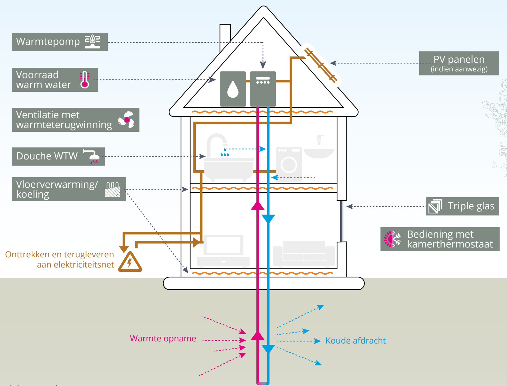
Schematisch overzicht energieconcept
